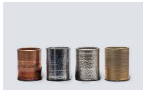
BAUTEIL: Zylinder WERKSTOFF: Kupfer, Titan, Edelstahl, Kupferlegierung / as-built AUSSENDURCHMESSER: 105 mm
